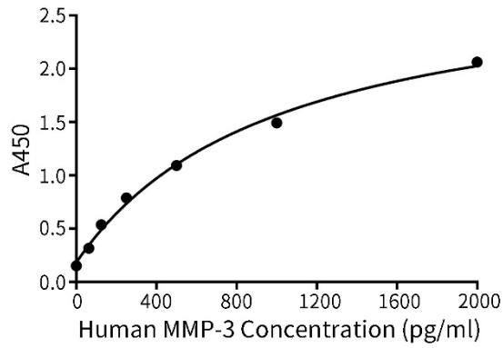
图3. Human Total MMP-3 ELISA Kit的标准曲线。实测数据会因实验条件、检测仪器等的不同而存在差异，图中数据仅供参考。
